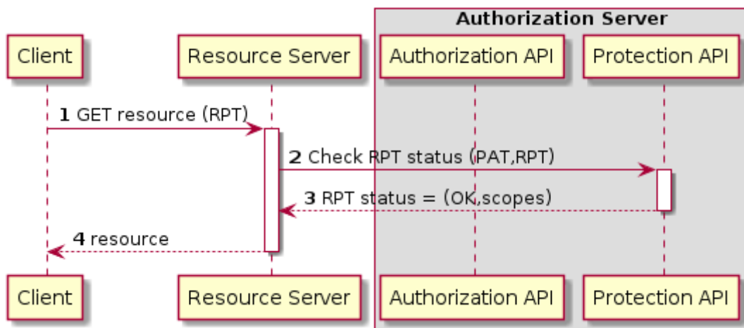
Figure 6. UMA Access Resource (Success)
