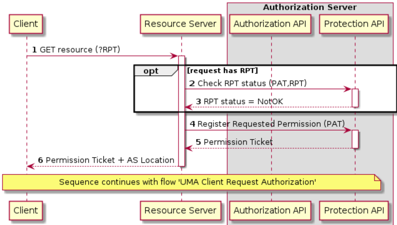
Figure 7. UMA Resource Server Register Permission
